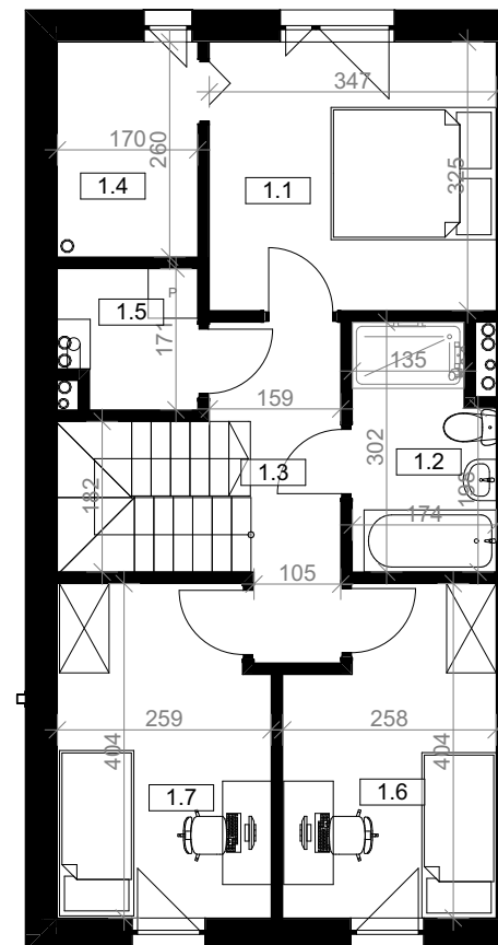
RZUT PIĘTRA
