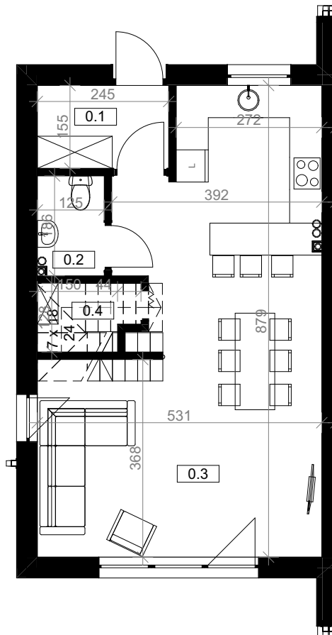
RZUT PARTERU
