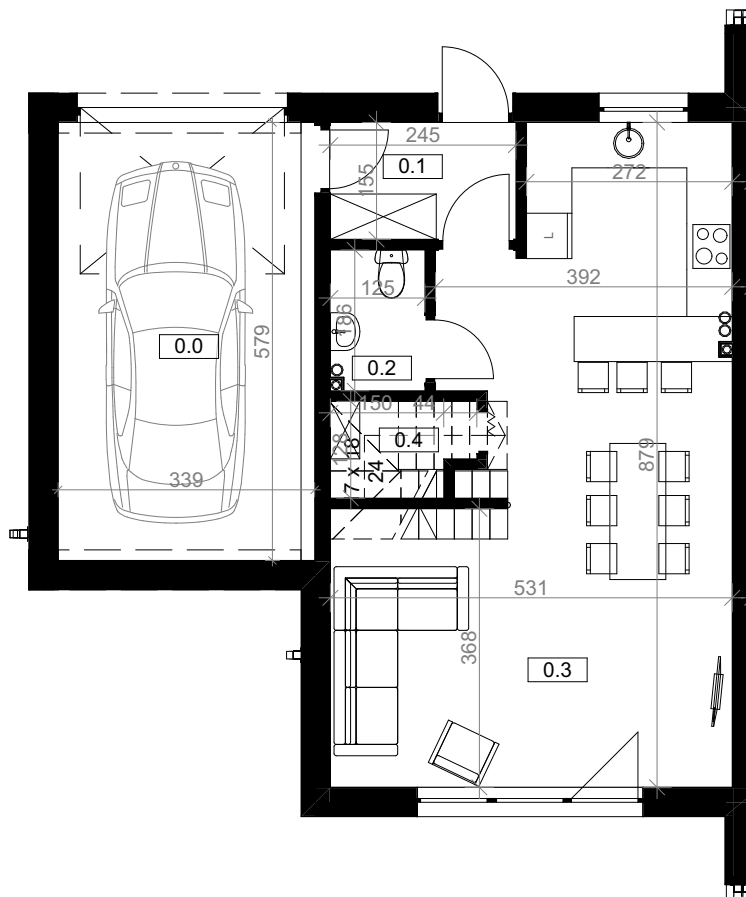
RZUT PARTERU
