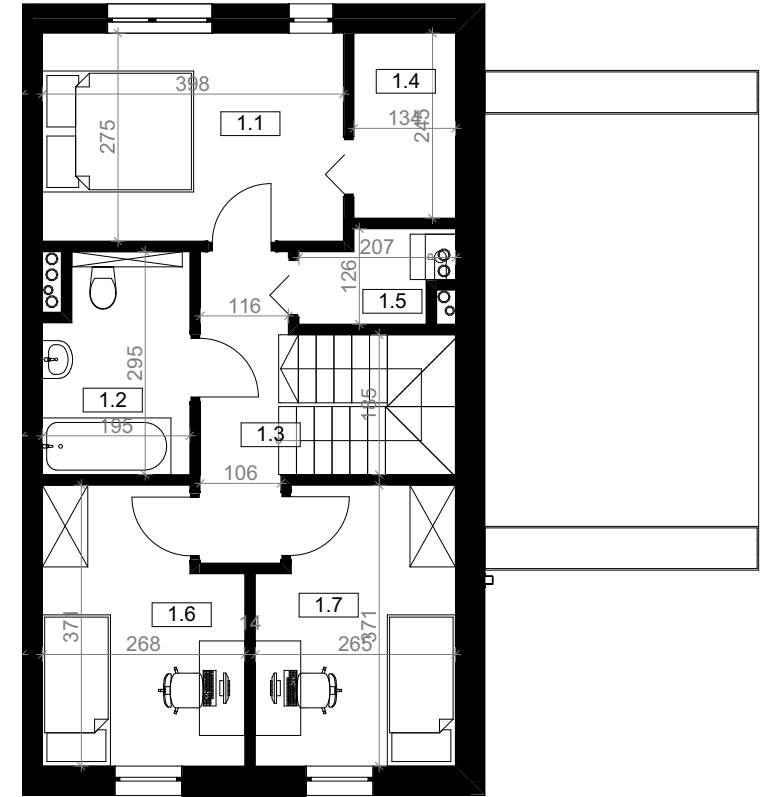
RZUT PIETRA
