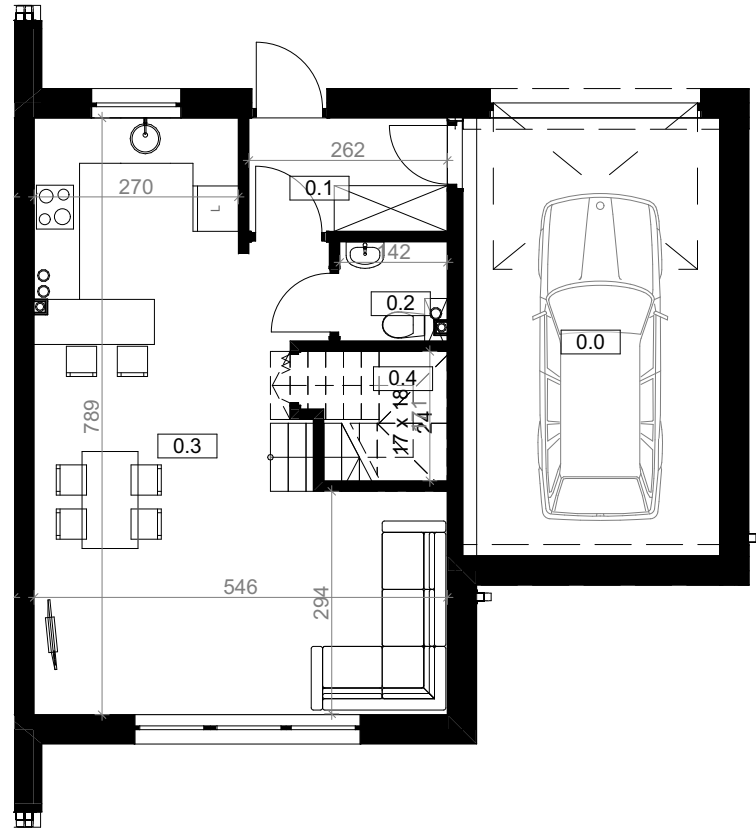
RZUT PARTERU
