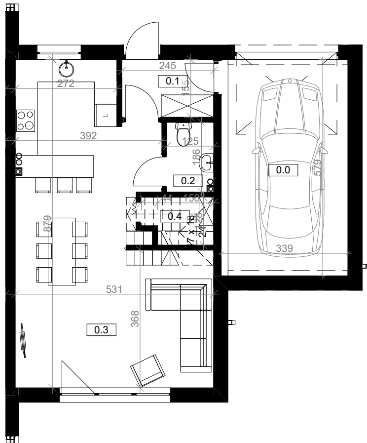
RZUT PARTERU
