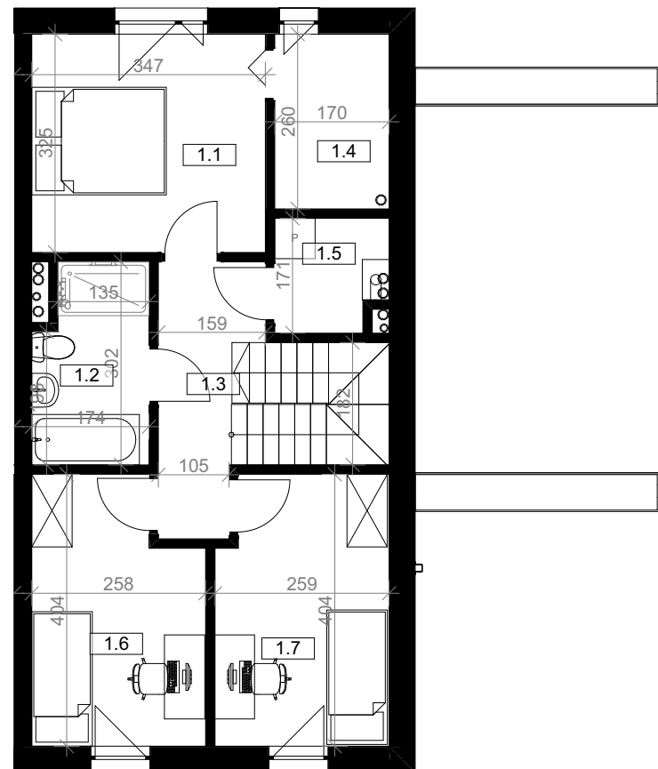
RZUT PIĘTRA
