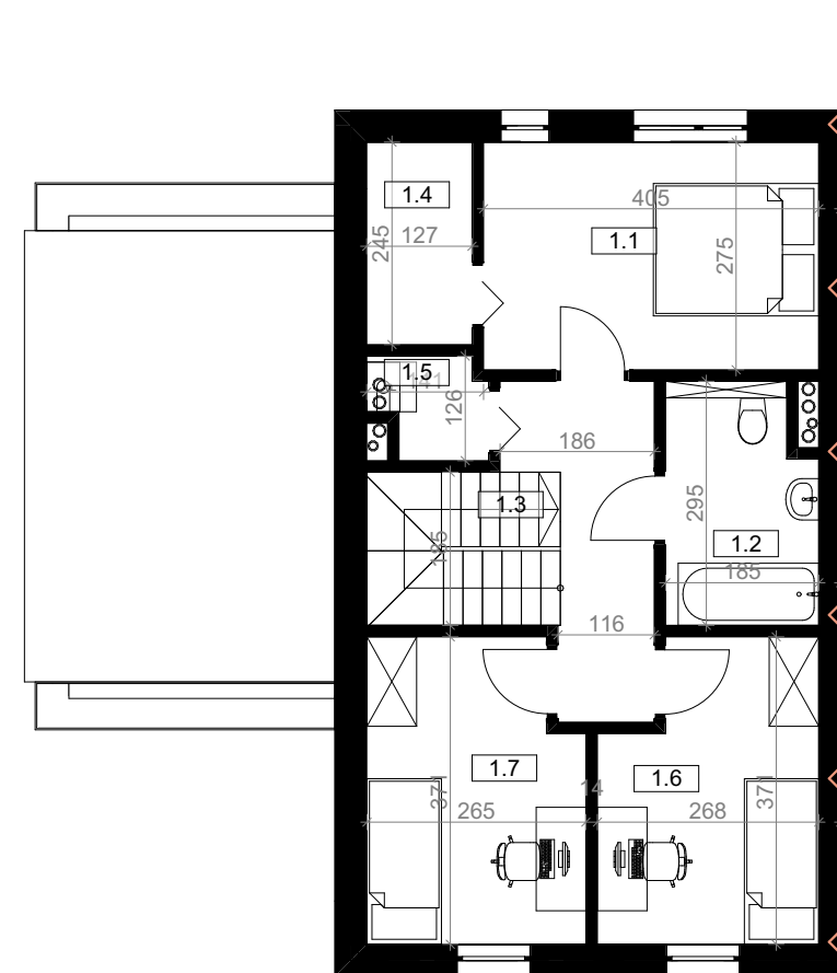
RZUT PIĘTRA
