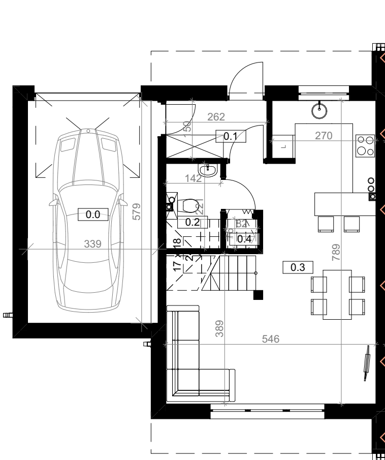
RZUT PARTERU
