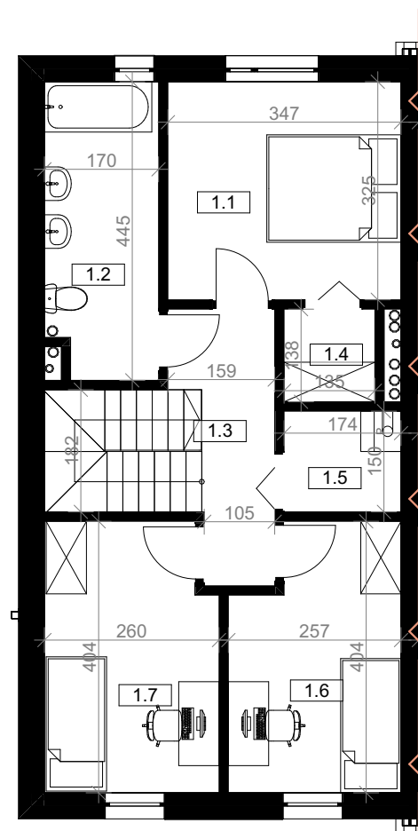
RZUT PIĘTRA
