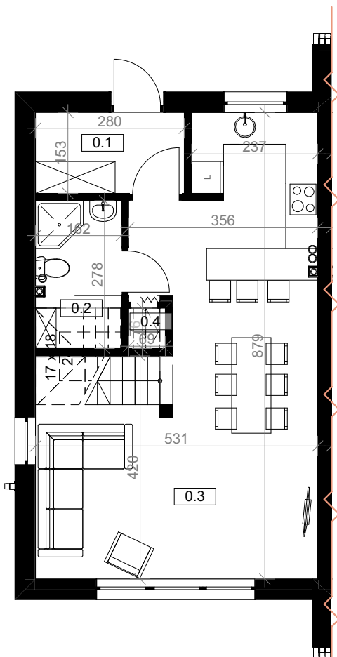
RZUT PARTERU
