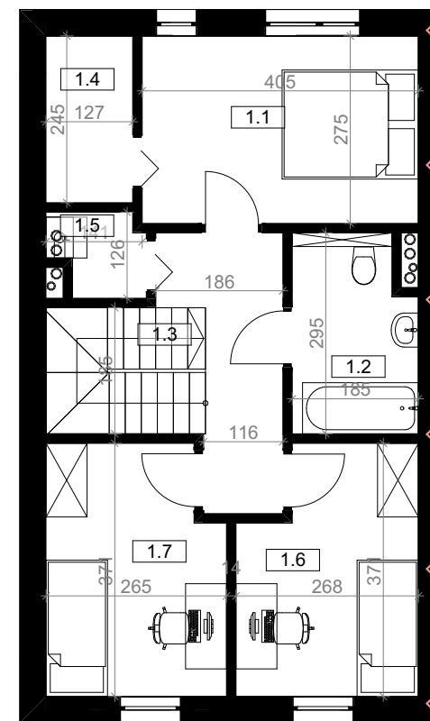
RZUT PIĘTRA
